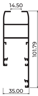
MARCO DE HOJA DE 90° ML4608
