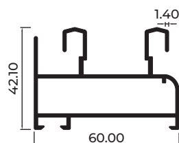
MARCO DOBLE CORREDIZA VL4601
