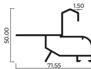
ADAPTADOR MARCO TRIPLE CORREDIZA ML4604
