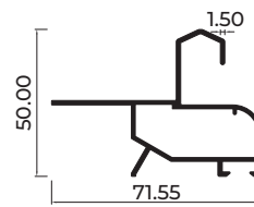
ADAPTADOR MARCO TRIPLE CORREDIZA ML4604
