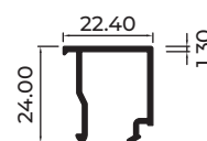
JUNQUILLO DE VIDRIO 6 MM Y 8 MM VL4608
