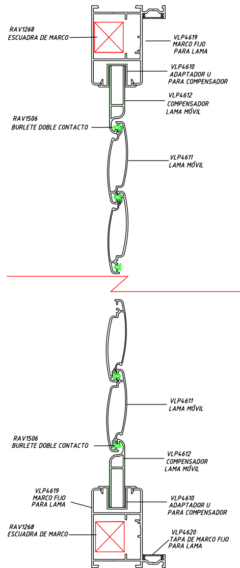
SECCIÓN VERTICAL
