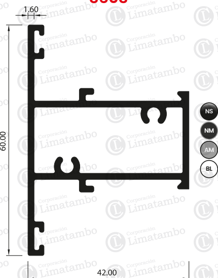
TRAVESAÑO
