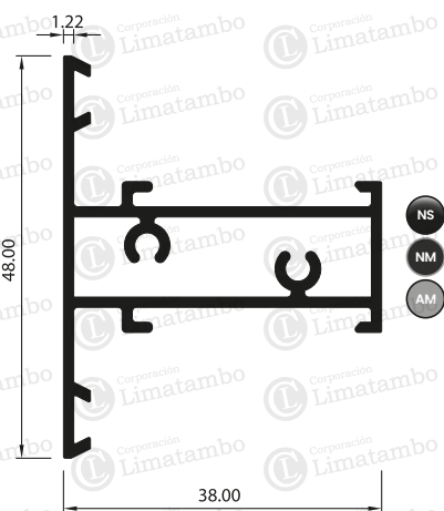
TRAVESAÑO
