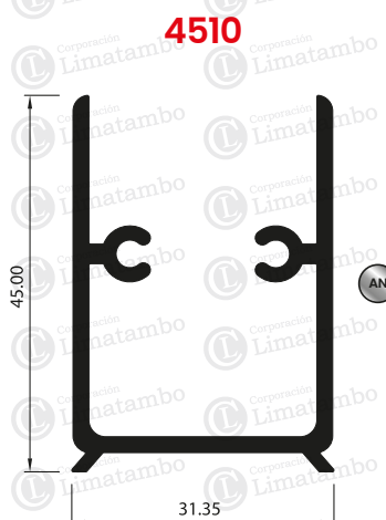
SOPORTE DE ARMADO
