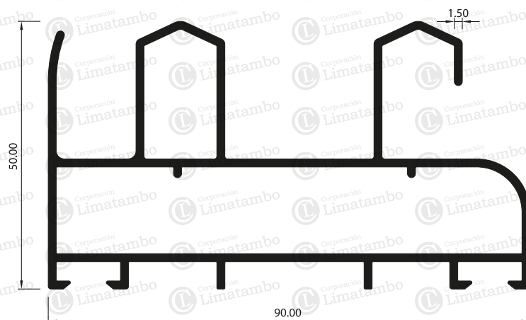
MARCO DOBLE CORREDIZA
