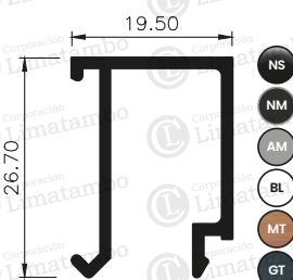
JUNQUILLO DE VIDRIO DE 10 MM Y 12 MM
