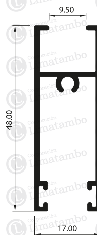
MARCO DE HOJA INFERIOR
