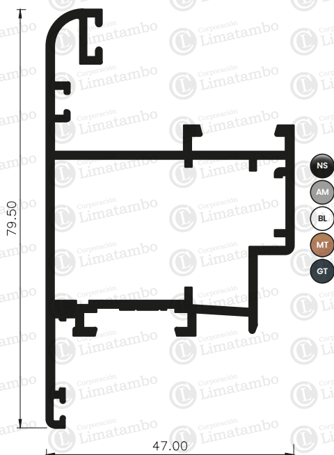
HOJA DE VENTANA APERTURA EXTERIOR PESADA
