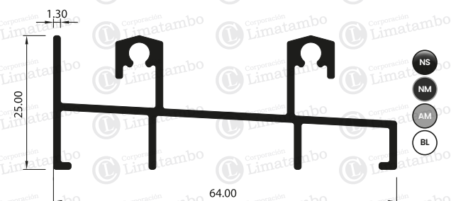
MARCO INFERIOR
