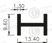
"H" PARA UNIÓN DE MARCOS
