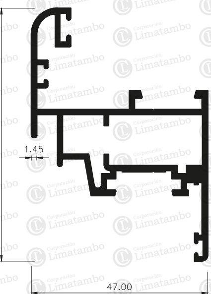
HOJA DE VENTANA APERTURA INTERIOR
