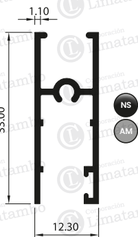
MARCO DE HOJA SUP. E INF. CORREDIZA
