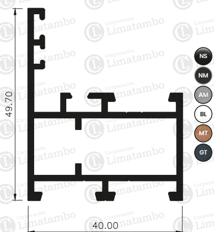
MARCO VENTANA
