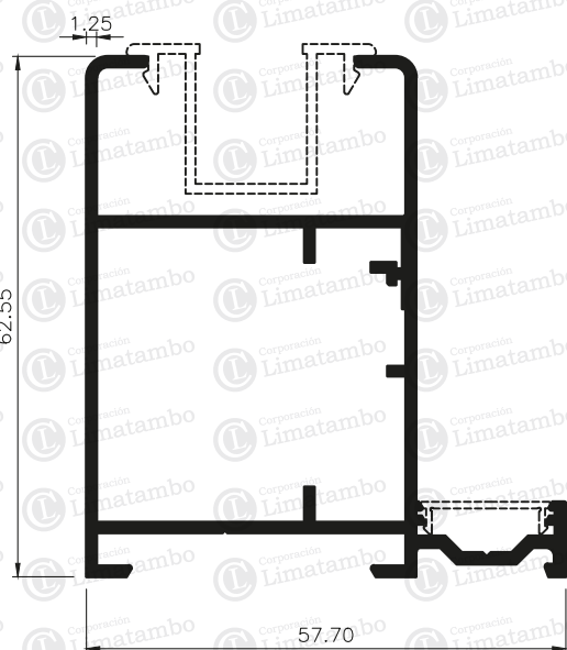
MARCO FIJO PARA LAMA
