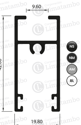
ZÓCALO DE HOJA SUPERIOR
