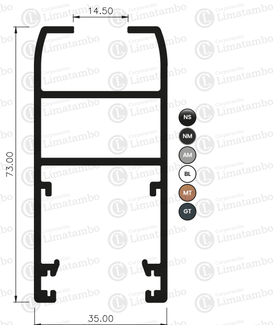
MARCO DE HOJA
