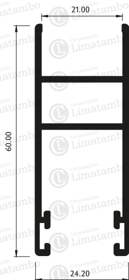
MARCO DE HOJA PARA INSULADO
