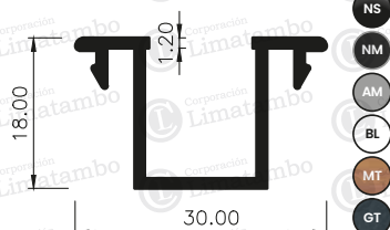
ADAPTADOR "U" PARA COMPENSADOR DE LAMA
