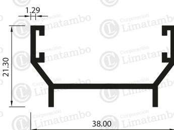
PERFIL ADAPTADOR
