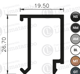
JUNQUILLO DE VIDRIO DE 10 MM Y 12 MM
