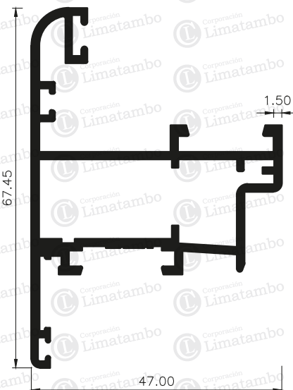
HOJA DE VENTANA APERTURA EXTERIOR
