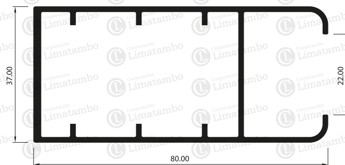
MONTANTE DE HOJA LIVIANA
