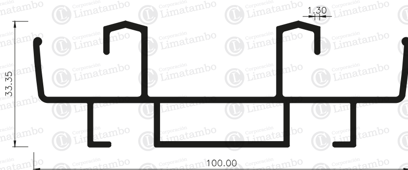
MARCO DOBLE CORREDIZA
