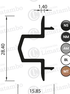
ADAPTADOR DE HOJA
