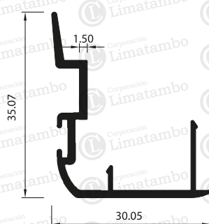
TRASLAPE
