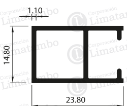
MARCO DE HOJA VERTICAL
