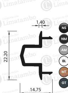
ADAPTADOR DE HOJA
