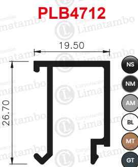
JUNQUILLO DE VIDRIO DE 10 MM Y 12 MM
