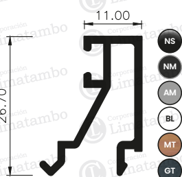
JUNQUILLO DE VIDRIO INSULADO
