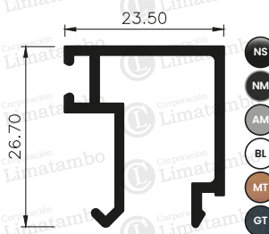
JUNQUILLO DE VIDRIO DE 6MM Y 8MM
