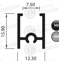
MARCO DE HOJA FIJO
