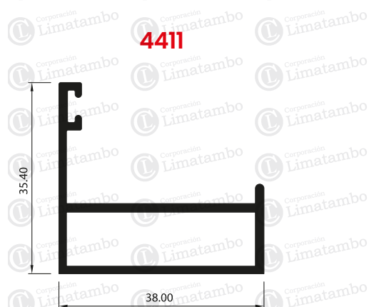
CONTRAMARCO DE VENTANA PROJ.
