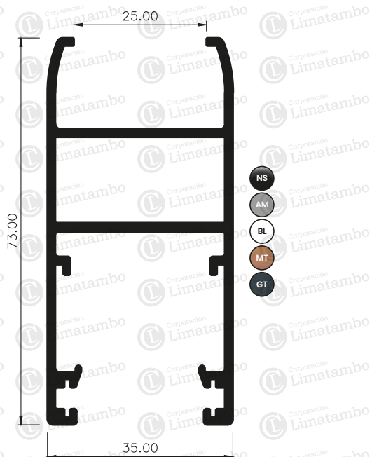
MARCO DE HOJA PARA INSULADO
