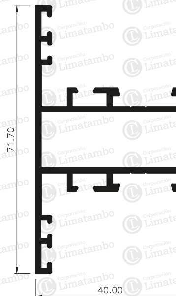
TRAVESAÑO DE VENTANA
