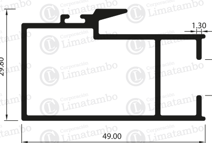
TRASLAPE DE HOJA
