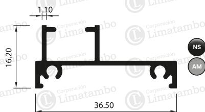
MARCO LATERAL FIJO
