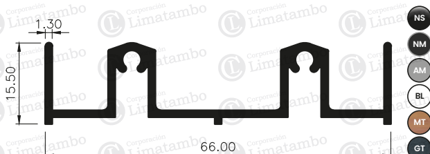
MARCO INFERIOR DE 15.5 MM
