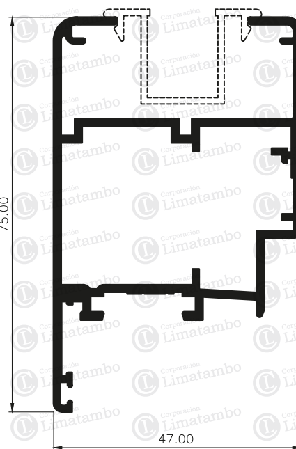
HOJA BATIENTE PARA LAMA MÓVIL
