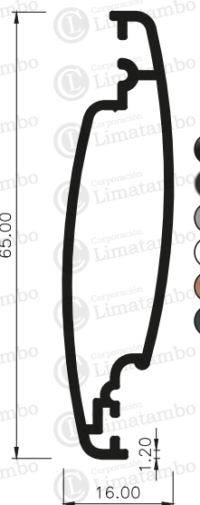
LAMA MÓVIL
