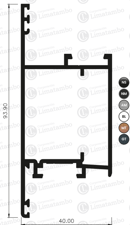
HOJA PUERTA APERTURA EXTERIOR
