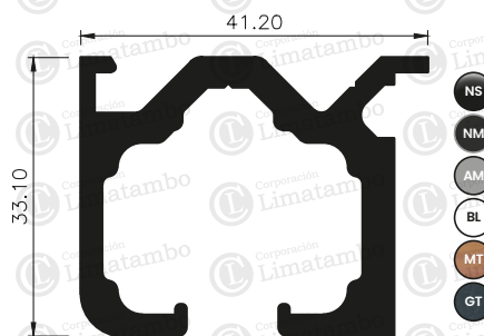
RIEL SUPERIOR PARA PLEGADIZA
