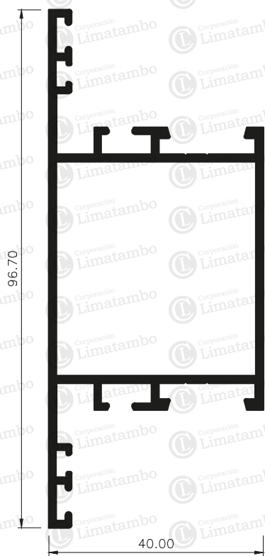
TRAVESAÑO DE PUERTA
