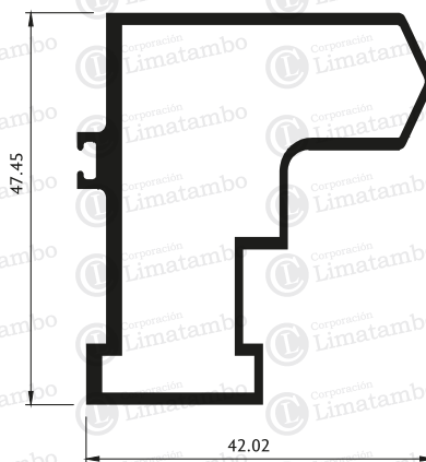
ADAPTADOR DE HOJA DE 90°
