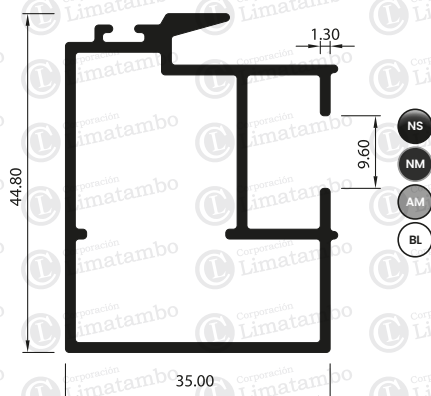
TRASLAPE DE HOJA
