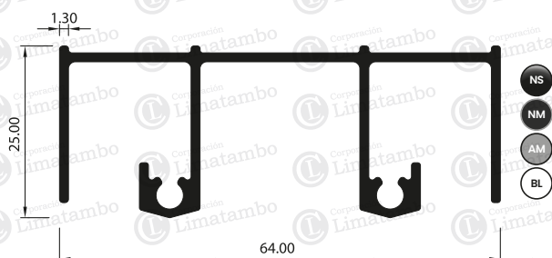
MARCO SUPERIOR
