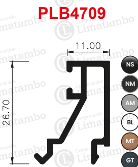
JUNQUILLO DE VIDRIO INSULADO
