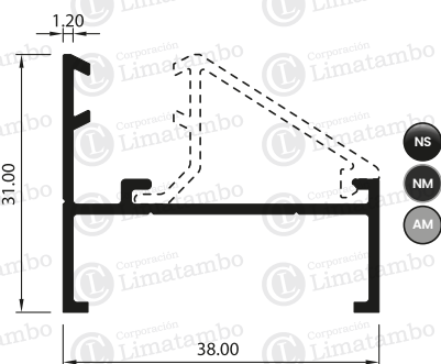
MARCO PROYECTANTE
