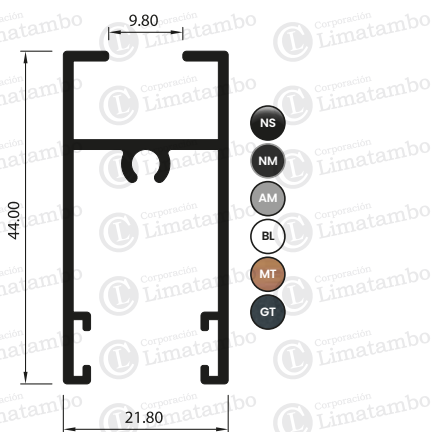
ZÓCALO DE HOJA SUPERIOR
