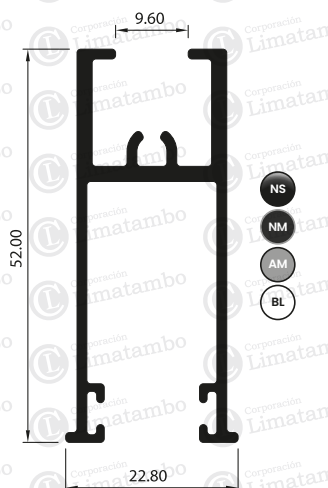
ZÓCALO DE HOJA INFERIOR
