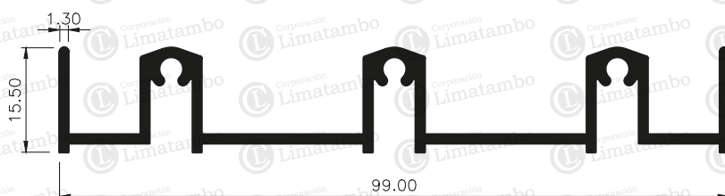
MARCO INFERIOR TRIPLE CARRIL DE 15.5 MM
