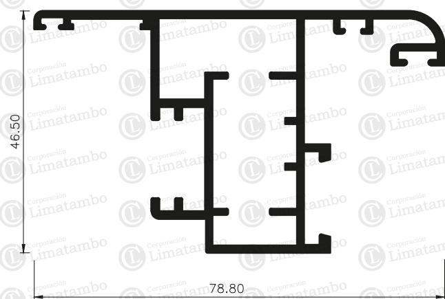
HOJA PIVOTANTE
