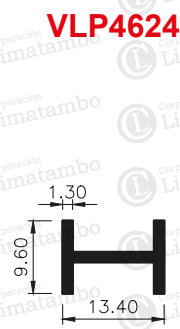
"H" PARA UNIÓN DE MARCOS
