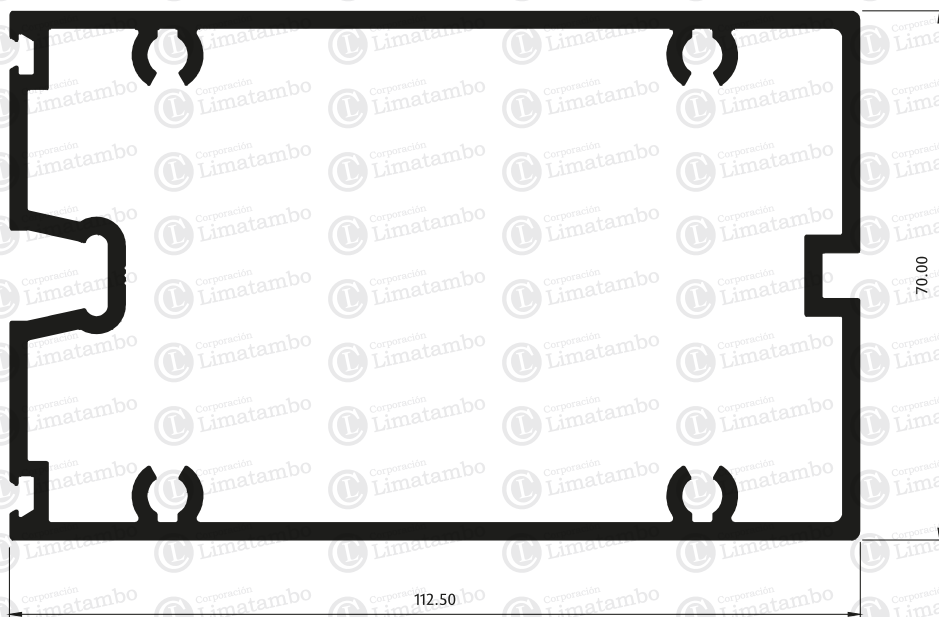
MONTANTE HORIZONTAL
