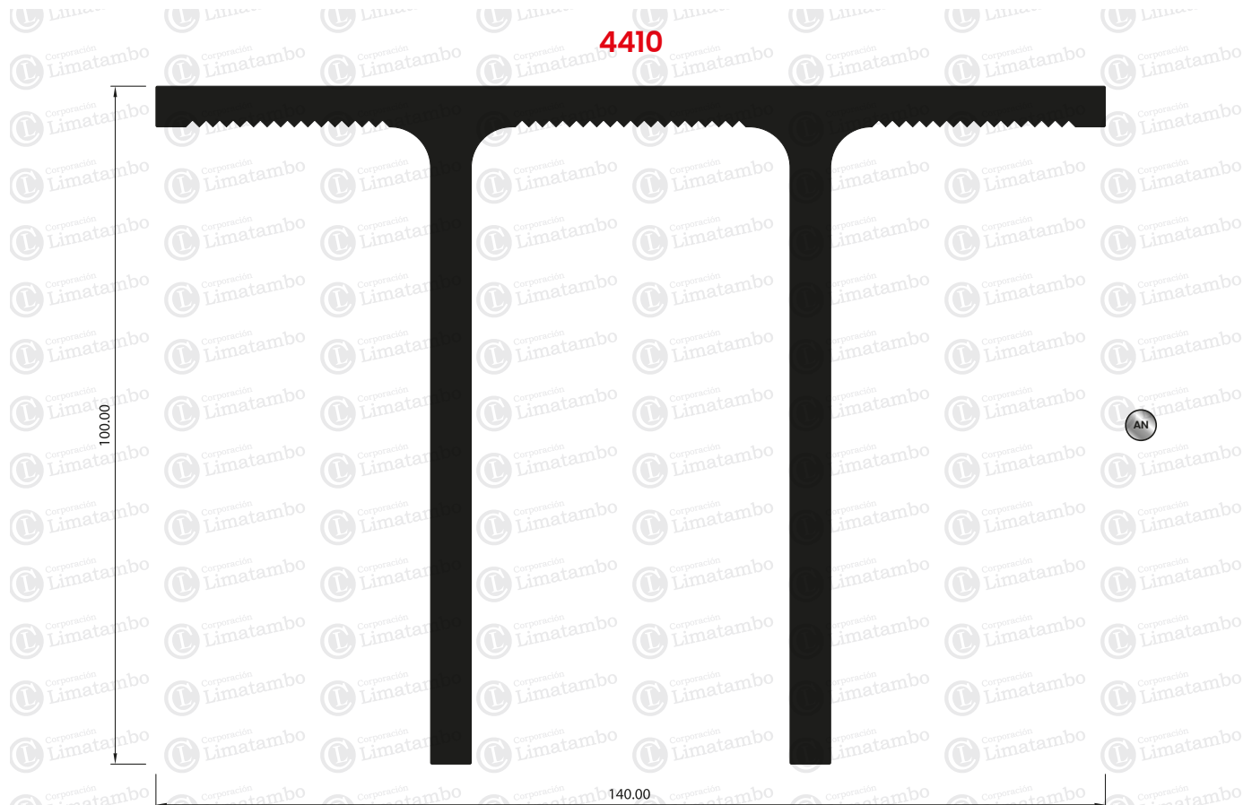
PERFIL ANCLAJE
