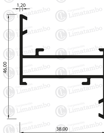
MARCO NAVE
