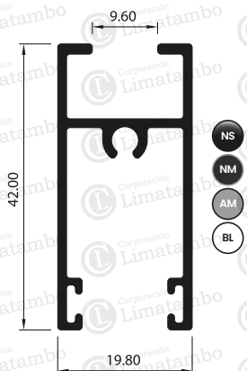
ZÓCALO DE HOJA SUPERIOR
