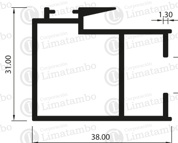
TRASLAPE
