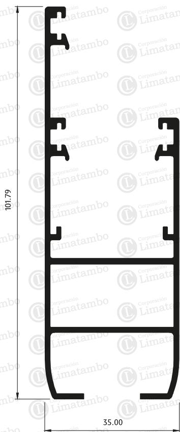
MARCO DE HOJA DE 90°
