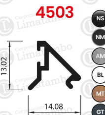
JUNQUILLO
