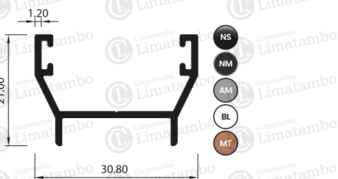
PERFIL ADAPTADOR DE HOJA
