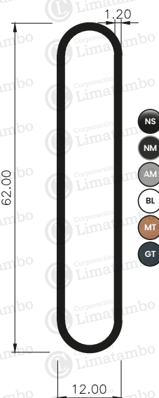
LAMA FIJA OVALINA
