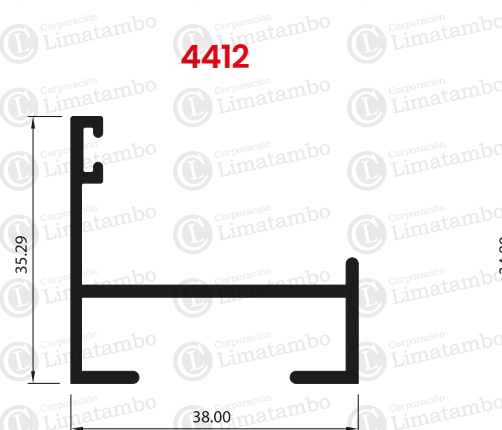
MARCO DE VENTANA PROJ.
