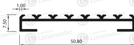
CORTAVIENTO
