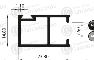
TRASLAPE DE HOJA
