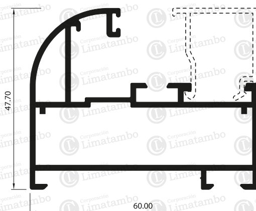
MARCO FIJO
