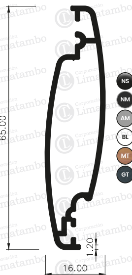
LAMA MÓVIL
