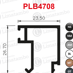
JUNQUILLO DE VIDRIO DE 6MM Y 8MM
