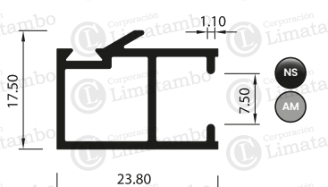
TRASLAPE DE HOJA
