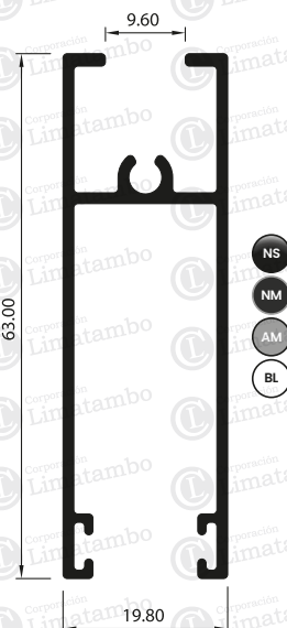
ZÓCALO DE HOJA INFERIOR
