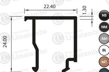
JUNQUILLO DE VIDRIO 6 MM Y 8 MM
