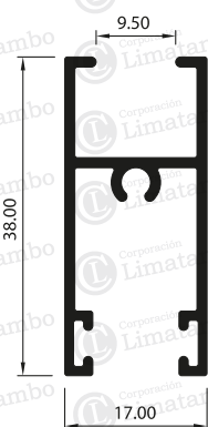
MARCO DE HOJA SUPERIOR
