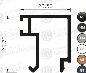
JUNQUILLO DE VIDRIO DE 6MM Y 8MM
