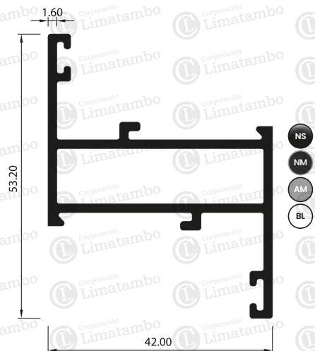
CONTRAMARCO
