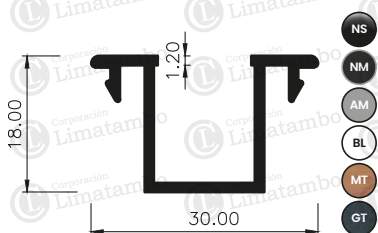
ADAPTADOR "U" PARA COMPENSADOR DE LAMA
