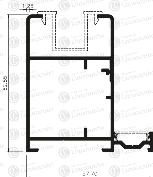
MARCO FIJO PARA LAMA
