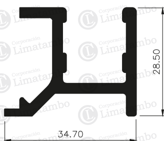
RIEL INFERIOR DE VENTANA PLEGADIZA
