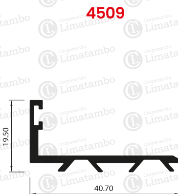
TOPE CON PORTAFELPA
