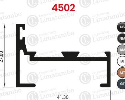
MARCO DE PUERTA
