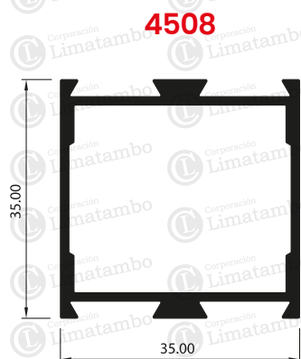
MARCO DE HOJA LIVIANA
