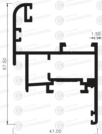
HOJA DE VENTANA APERTURA INTERIOR
