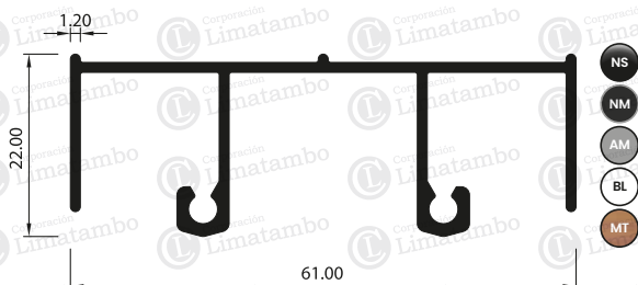
MARCO SUPERIOR
