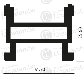
CALZO DE ADAPTADOR DE HOJA DE 90°
