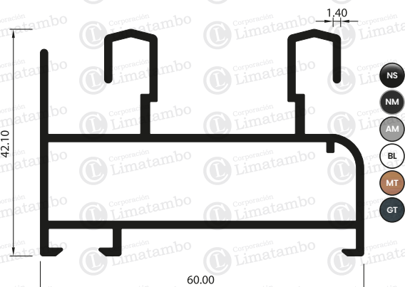
MARCO DOBLE CORREDIZA
