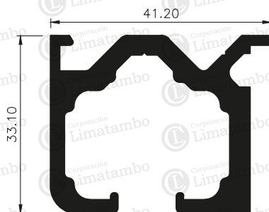
RIEL SUPERIOR PARA PLEGADIZA
