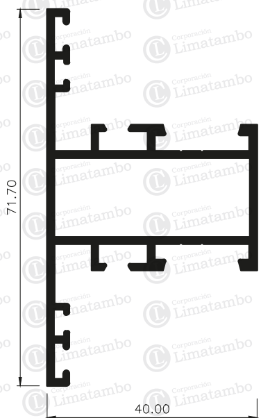
TRAVESAÑO DE VENTANA
