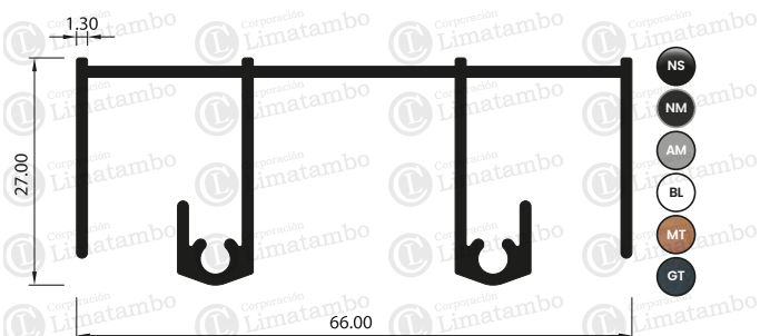
MARCO SUPERIOR
