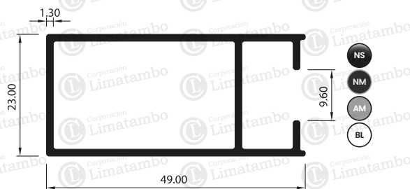
MARCO DE HOJA LATERAL
