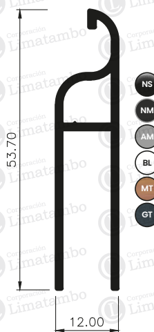
COMPENSADOR LAMA MÓVIL
