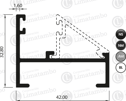
MARCO PROYECTANTE
