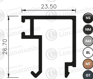
JUNQUILLO DE VIDRIO DE 6MM Y 8MM
