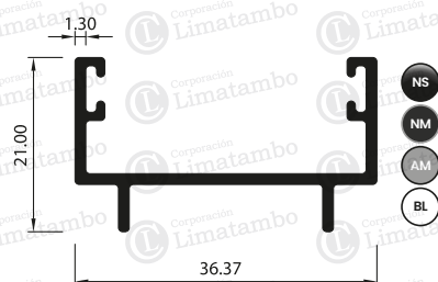
PERFIL ADAPTADOR DE HOJA
