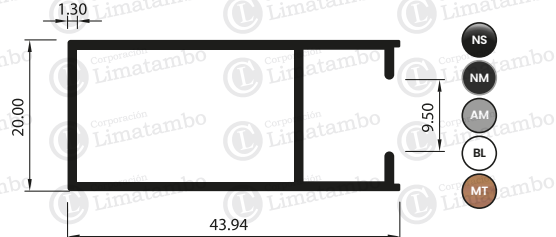
MARCO DE HOJA LATERAL
