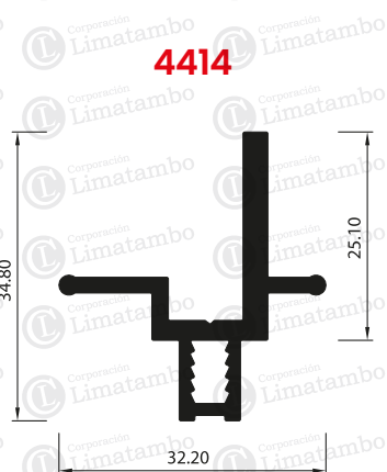
CLIP DE SUJECIÓN HORIZONTAL PARA INSULADOS
