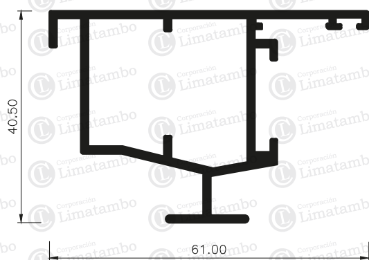
INVERSOR HOJA PIVOTANTE
