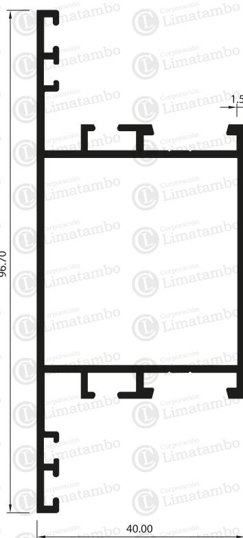
TRAVESAÑO DE PUERTA
