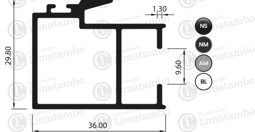
TRASLAPE DE HOJA
