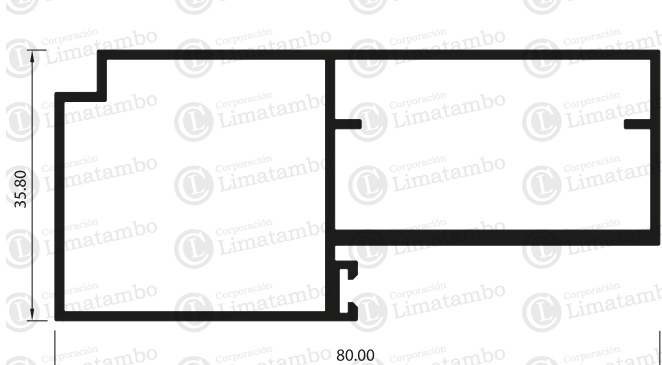
MARCO PUERTA
