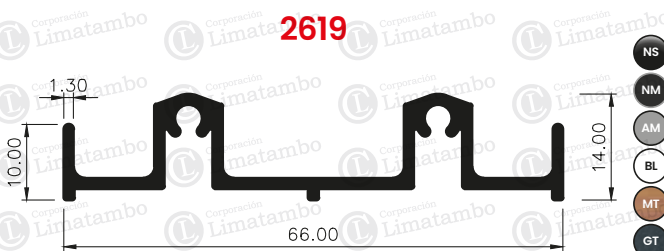
MARCO INFERIOR PARA PISO LAMINADO 10 MM
