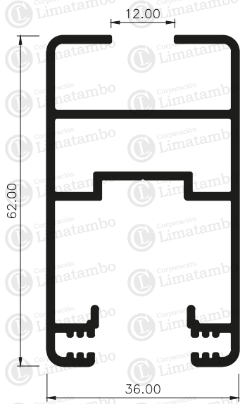
MARCO DE HOJA
