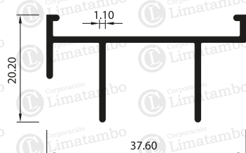
MARCO SUP. DOBLE CORREDIZA
