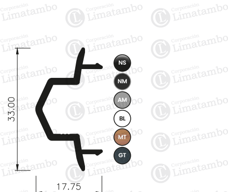
ADAPTADOR DE HOJA
