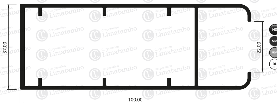
MONTANTE DE HOJA PESADA
