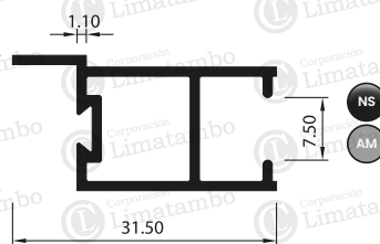
MARCO DE HOJA ENCUENTRO CORREDIZAS
