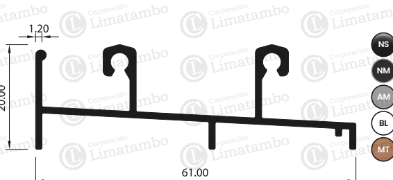
MARCO INFERIOR
