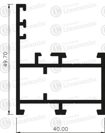
MARCO VENTANA
