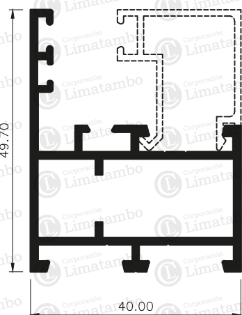
MARCO VENTANA
