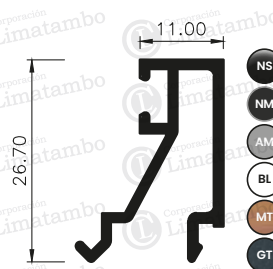
JUNQUILLO DE VIDRIO INSULADO
