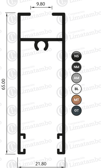
ZÓCALO DE HOJA INFERIOR
