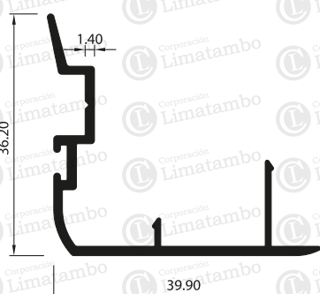
TRASLAPE DE HOJA
