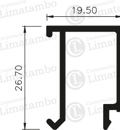
JUNQUILLO DE VIDRIO DE 10 MM Y 12 MM
