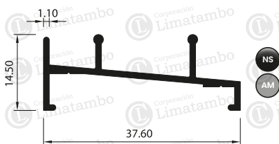
MARCO INF. DOBLE CORREDIZA
