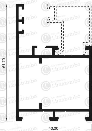
MARCO PUERTA
