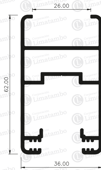
MARCO DE HOJA PARA INSULADO
