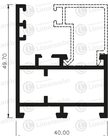
MARCO VENTANA
