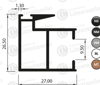
TRASLAPE
