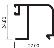
JUNQUILLO 8MM MBL4608
