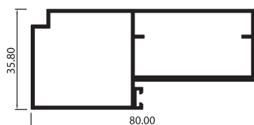
MARCO PUERTA MBL4600
