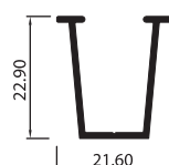
ADAPTADOR CRISTAL SIMPLE MBL4609
