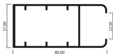
MONTANTE DE HOJA LIVIANA MBL4603
