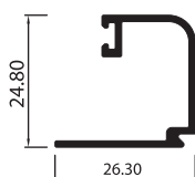
JUNQUILLO 18MM MBL4606
