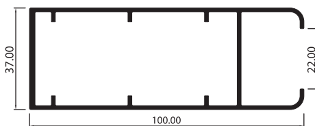
MONTANTE DE HOJA PESADA MBL4604
