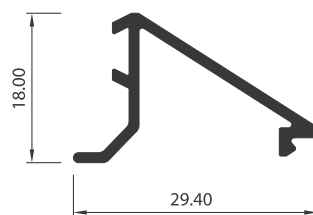
JUNQUILLO ALN 177
