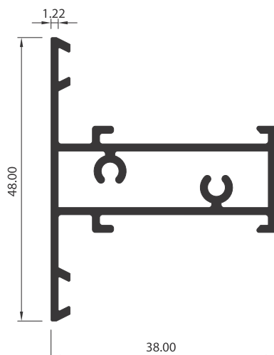
TRAVESAÑO ALN 292
