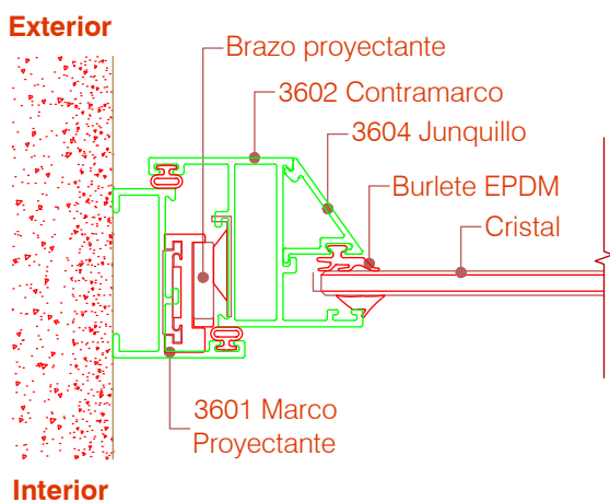
Det. 01
