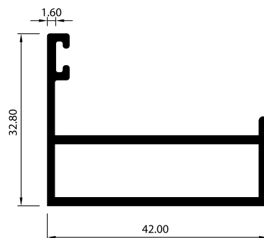
CONTRAMARCO MÓVIL PARA PROYECTANTE 3606
