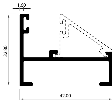
MARCO PROYECTANTE 3601
