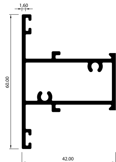
TRAVESAÑO 3603
