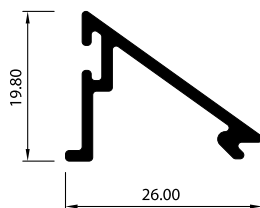
JUNQUILLO 3604
