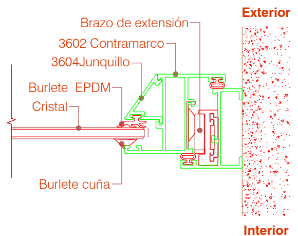
Det. 02
