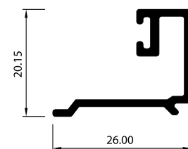
JUNQUILLO PARA INSULADO 3607
