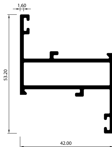
CONTRAMARCO 3602
