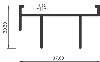
MARCO SUP. DOBLE CORREDIZA 3501
