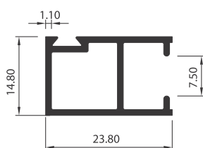
TRASLAPE DE HOJA 3510
