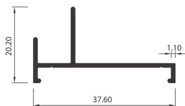
MARCO SUP. FIJO CORREDIZA 3502
