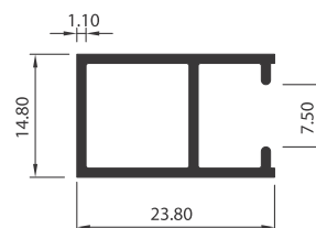
MARCO HOJA LATERAL 3509
