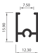
MARCO HOJA FIJO 3511
