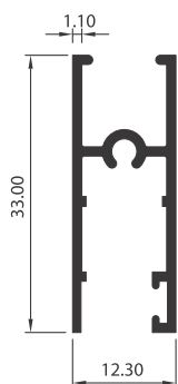
MARCO DE HOJA 3507
