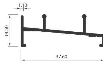
MARCO INF. DOBLE CORREDIZA 3503
