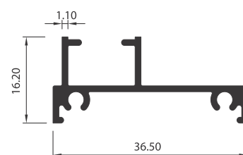
MARCO LATERAL FIJO 3506
