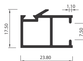
TRASLAPE DE HOJA 3513
