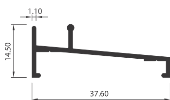
MARCO INF. FIJO CORREDIZA 3504
