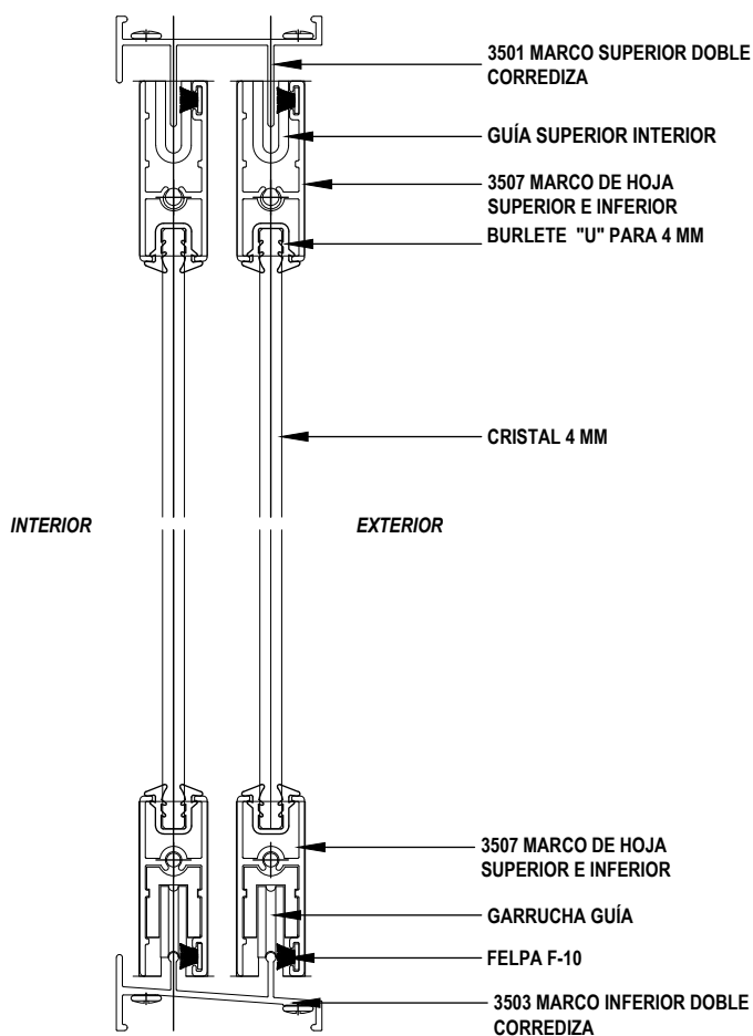
CORTE ①-①
