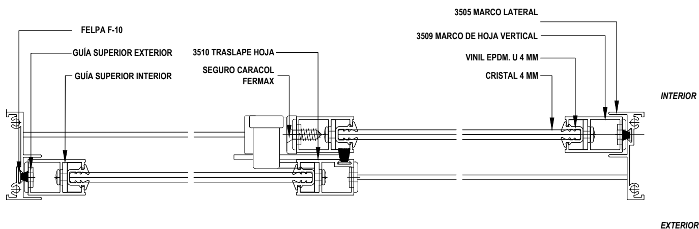
CORTE ②-②
