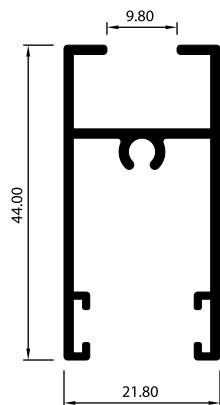
ZÓCALO SUPERIOR 2604
