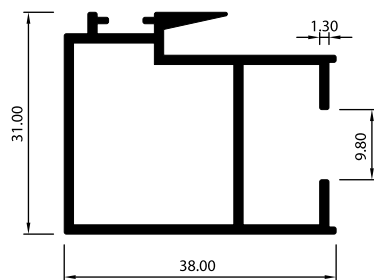
TRASLAPE 2607
