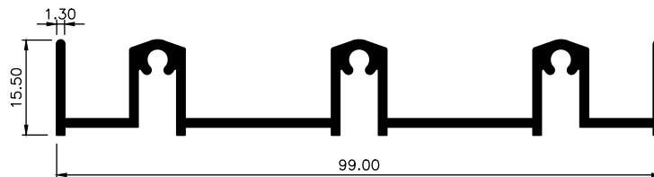
MARCO INFERIOR TRIPLE CARRIL DE 15.5 MM 2613
