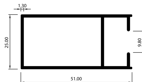
MARCO LATERAL DE HOJA 2610
