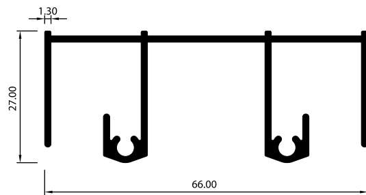
RIEL SUPERIOR 2601
