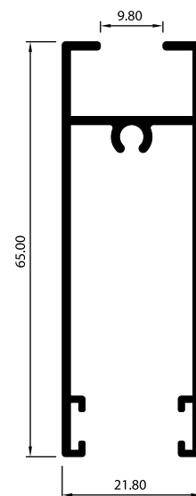
ZÓCALO INFERIOR 2605
