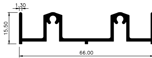
MARCO INFERIOR DE 15.5 MM 2612
