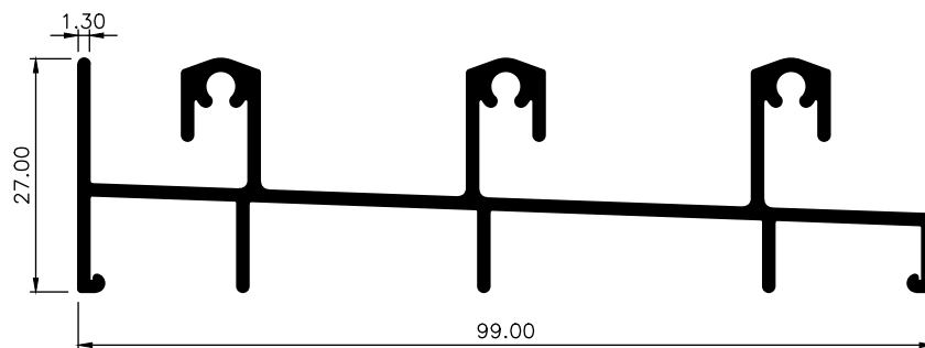
MARCO INFERIOR TRIPLE CARRIL 2615
