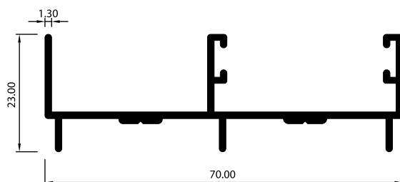
MARCO LATERAL 2609
