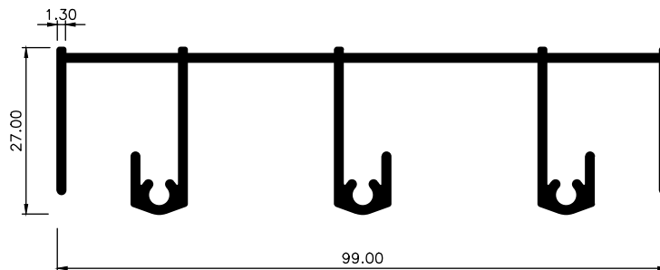
MARCO SUPERIOR TRIPLE CARRIL 2614
