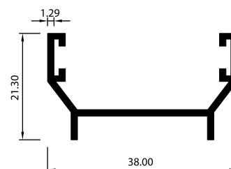
PERFIL ADAPTADOR 2608
