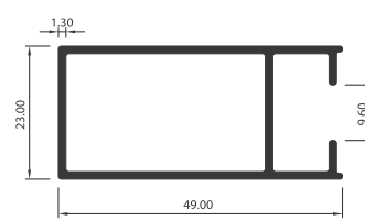
MARCO DE HOJA LATERAL VL4206
