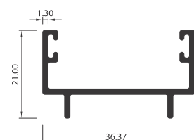
PERFIL ADAPTADOR DE HOJA ML4214
