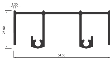
MARCO SUPERIOR VL4201
