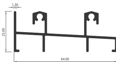
MARCO INFERIOR VL4202
