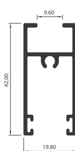
ZÓCALO DE HOJA SUPERIOR VL4209
