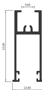
ZÓCALO DE HOJA INFERIOR VL4210
