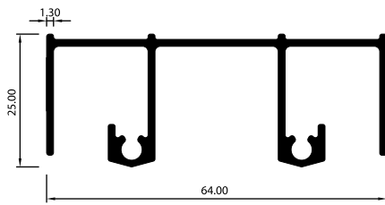
MARCO SUPERIOR VL4201
