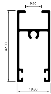
ZÓCALO DE HOJA SUPERIOR VL4209
