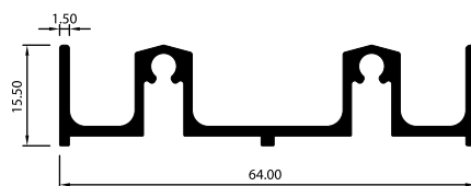
MARCO INFERIOR ML4205
