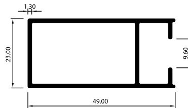
MARCO DE HOJA LATERAL VL4206
