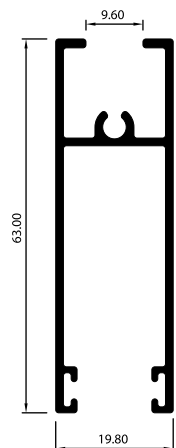
ZÓCALO DE HOJA INFERIOR ML4201
