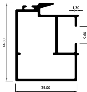
TRASLAPE DE HOJA ML4204
