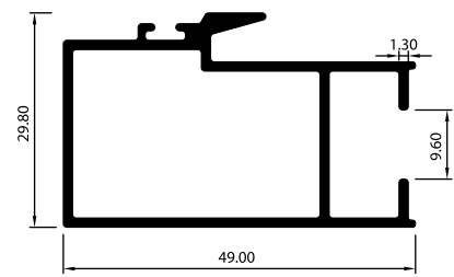
TRASLAPE DE HOJA ML4203
