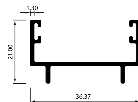
PERFIL ADAPTADOR DE HOJA ML4214
