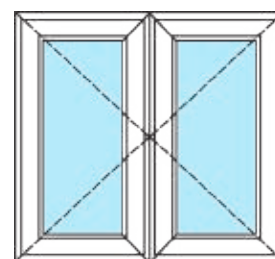
2 Hojas Apertura Exterior VLP46
