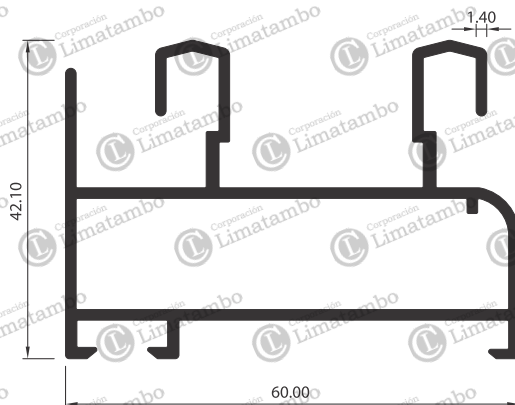
MARCO DOBLE CORREDIZA
