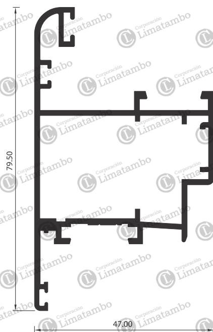
HOJA DE VENTANA APERTURA EXTERIOR PESADA
