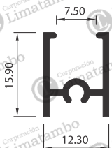
MARCO DE HOJA FIJO
