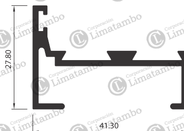
MARCO DE PUERTA
