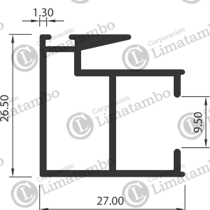
TRASLAPE
