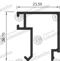
JUNQUILLO DE VIDRIO DE 6MM Y 8MM
