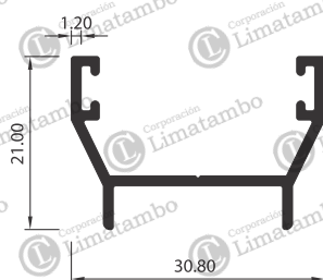
PERFIL ADAPTADOR DE HOJA
