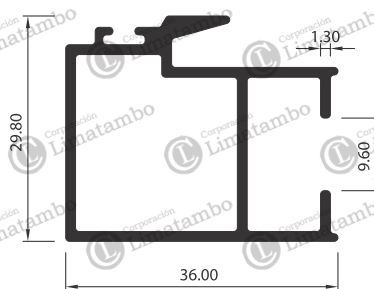
TRASLAPE DE HOJA
