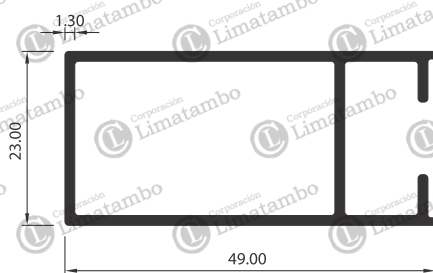
MARCO DE HOJA LATERAL
