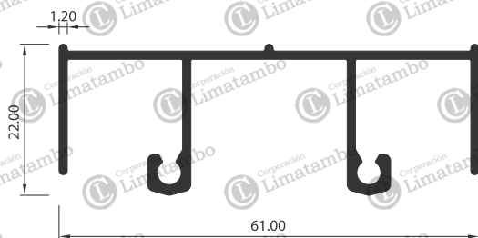
MARCO SUPERIOR
