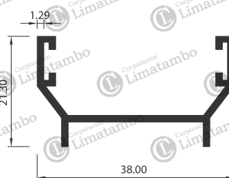
PERFIL ADAPTADOR
