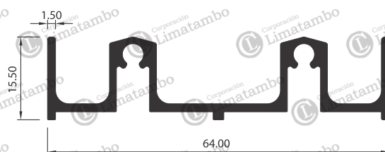
MARCO INFERIOR
