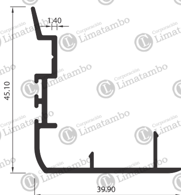
TRASLAPE DE HOJA
