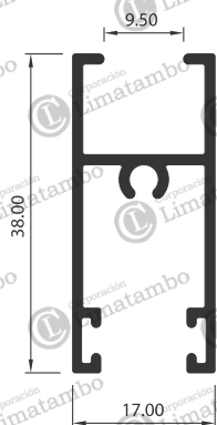
MARCO DE HOJA SUPERIOR
