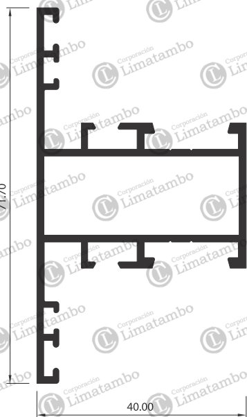
TRAVESAÑO DE VENTANA
