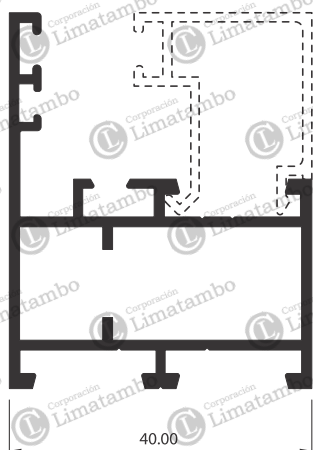
MARCO VENTANA
