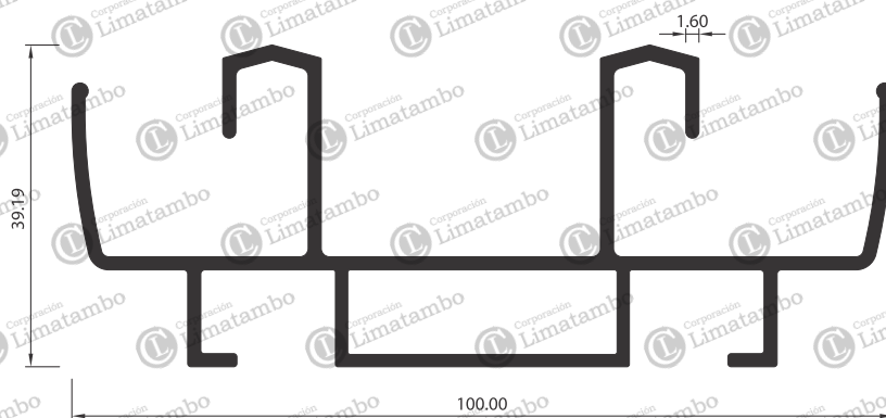
MARCO DOBLE CORREDIZA
