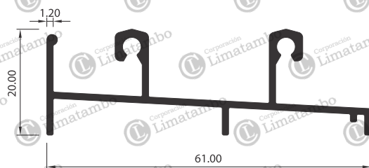
MARCO INFERIOR
