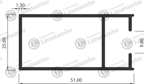
MARCO LATERAL DE HOJA
