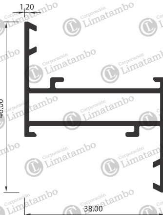
MARCO NAVE
