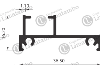
MARCO LATERAL FIJO
