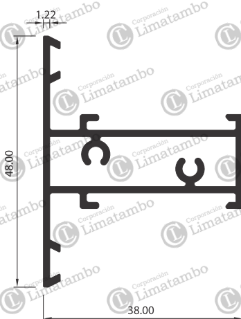
TRAVESAÑO
