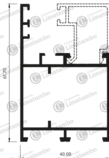
MARCO PUERTA
