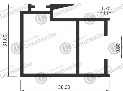
TRASLAPE
