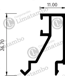
JUNQUILLO DE VIDRIO INSULADO
