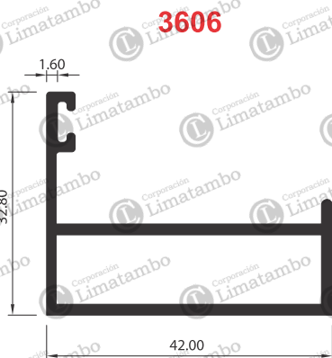
MARCO
