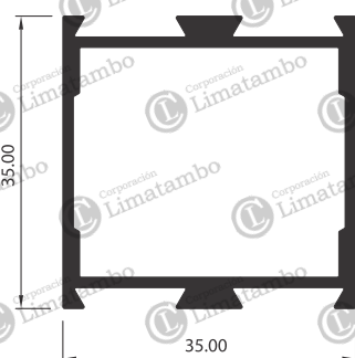
MARCO DE HOJA LIVIANA
