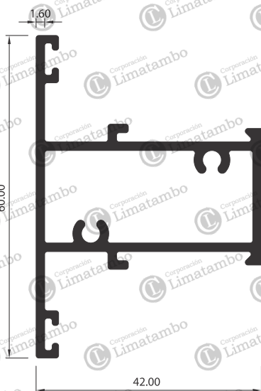
TRAVESAÑO
