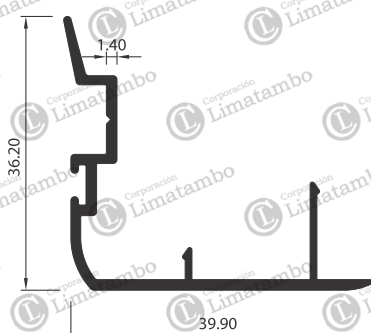
TRASLAPE DE HOJA
