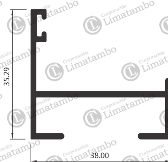
MARCO DE VENTANA PROJ.
