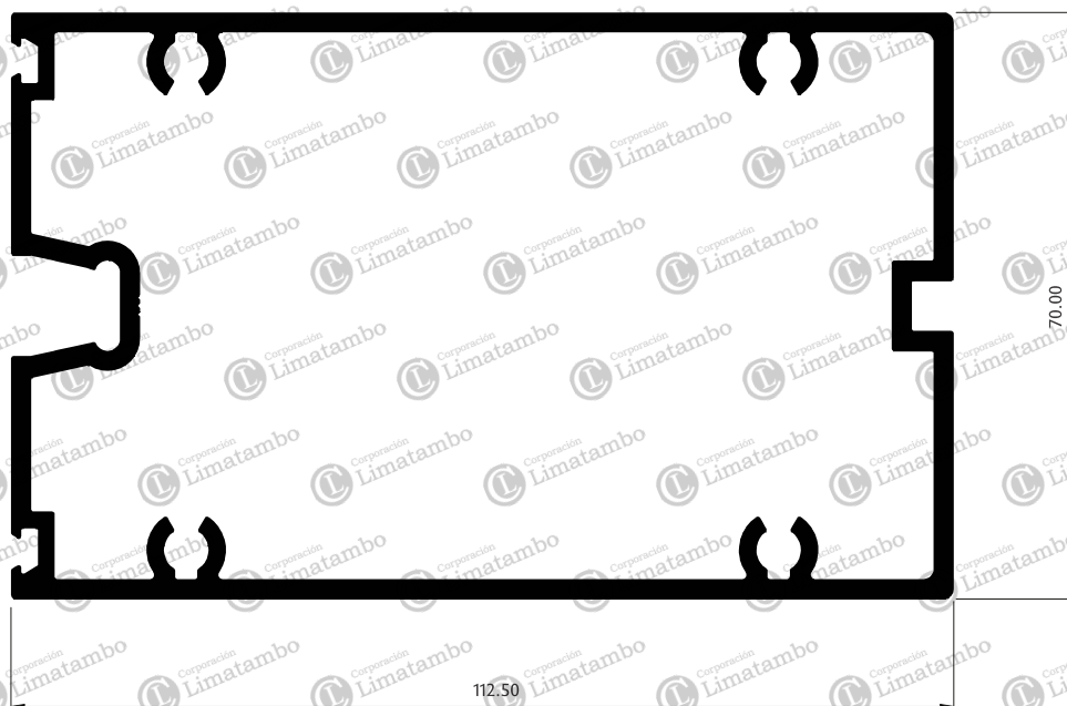
MONTANTE HORIZONTAL
