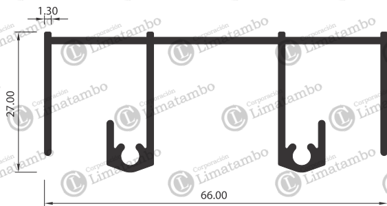
MARCO SUPERIOR
