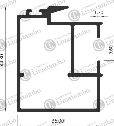
TRASLAPE DE HOJA
