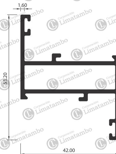
CONTRAMARCO
