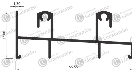
MARCO INFERIOR
