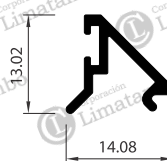
JUNQUILLO
