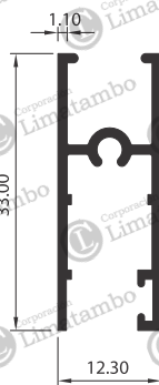
MARCO DE HOJA SUP. E INF. CORREDIZA
