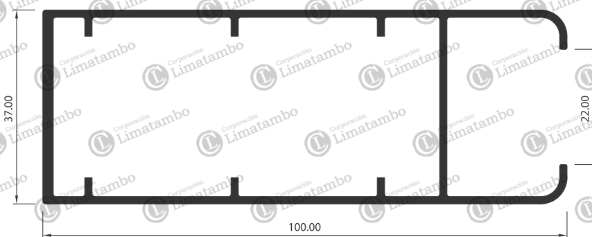
MONTANTE DE HOJA PESADA
