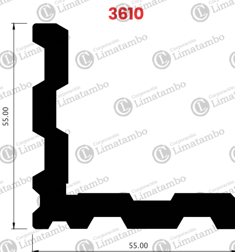
ÁNGULO RANURADO
