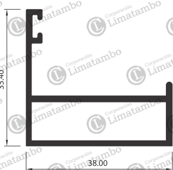
CONTRAMARCO DE VENTANA PROJ.
