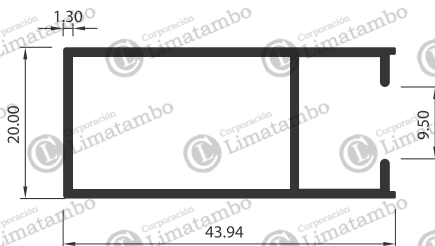
MARCO DE HOJA LATERAL
