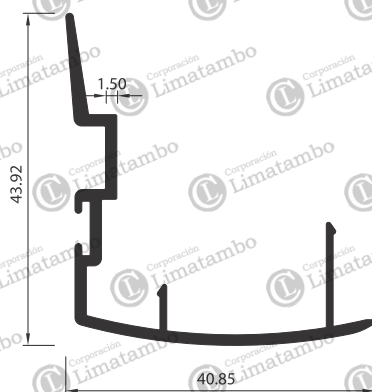
TRASLAPE
