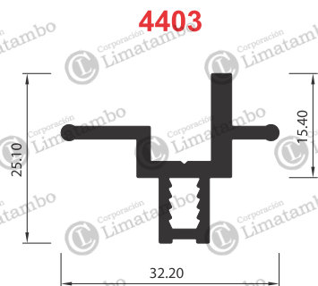
CLIP DE SUJECIÓN HORIZONTAL
