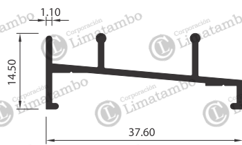
MARCO INF. DOBLE CORREDIZA
