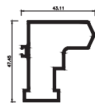
ADAPTADOR DE HOJA DE 90° ML4610
