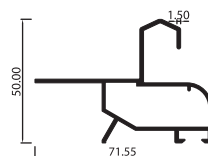
ADAPTADOR MARCO TRIPLE CORREDIZA ML4604
