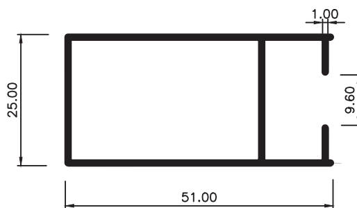
MARCO DE HOJA LATERAL
