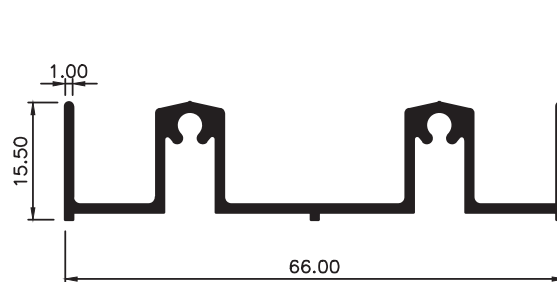
MARCO INFERIOR EMPOTRABLE
