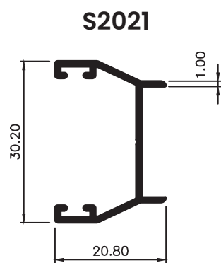
PERFIL ADAPTADOR DE HOJA
