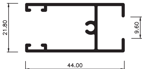
MARCO DE HOJA SUPERIOR
