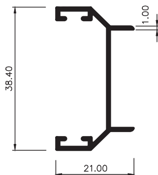
PERFIL ADAPTADOR DE HOJA
