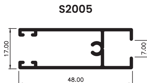
MARCO DE HOJA INFERIOR
