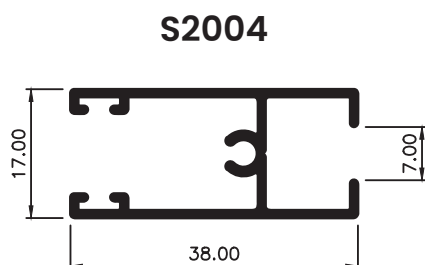
MARCO DE HOJA SUPERIOR
