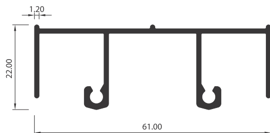
RIEL SUPERIOR 1901
