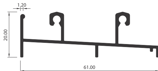
RIEL INFERIOR 1902
