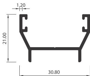
PERFIL ADAPTADOR 1908
