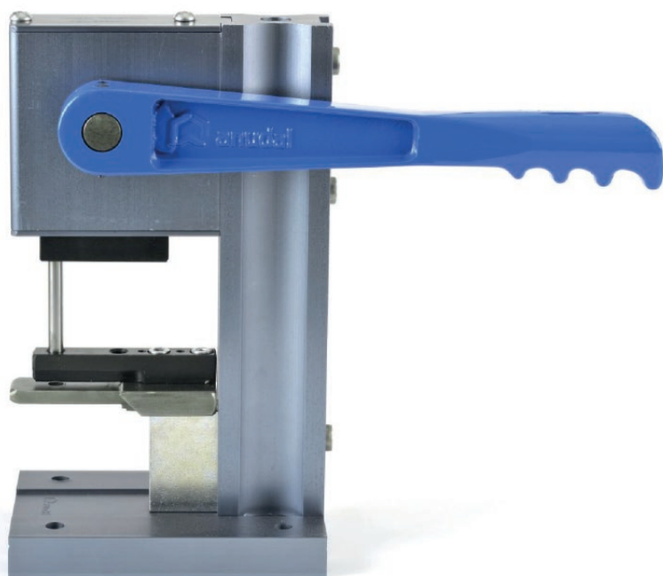
Punzadora manual pivote Cód: RAF000639 (Para serie VL46, ML46 y VL48)
