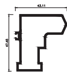
ADAPTADOR DE HOJA DE 90° ML4610
