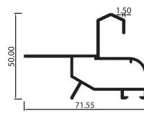
ADAPTADOR MARCO TRIPLE CORREDIZA ML4604
