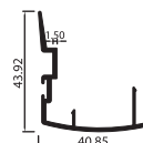
TRASLAPE ML4603
