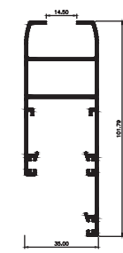
MARCO DE HOJA DE 90° ML4608
