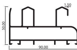
MARCO DOBLE CORREDIZA ML4601
