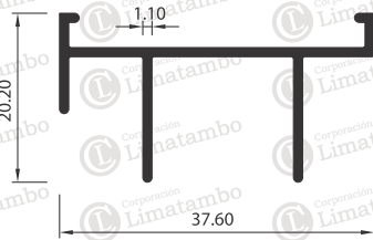
MARCO SUP. DOBLE CORREDIZA
