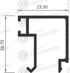
JUNQUILLO DE VIDRIO DE 6MM Y 8MM
