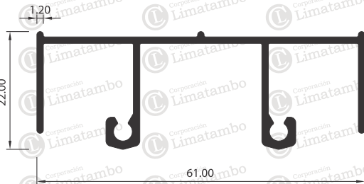
MARCO SUPERIOR
