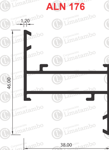
MARCO NAVE
