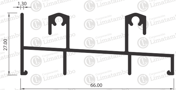
MARCO INFERIOR
