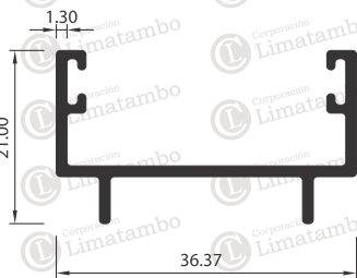
PERFIL ADAPTADOR DE HOJA
