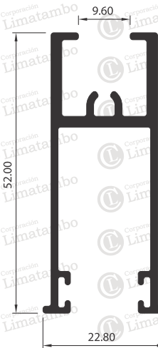
ZÓCALO DE HOJA INFERIOR
