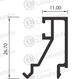
JUNQUILLO DE VIDRIO INSULADO
