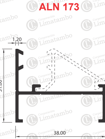
MARCO PROYECTANTE
