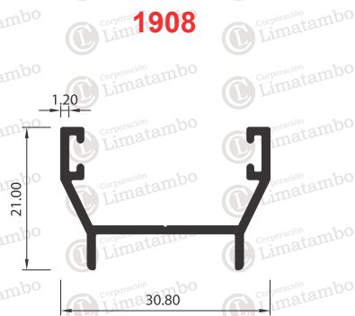
PERFIL ADAPTADOR DE HOJA
