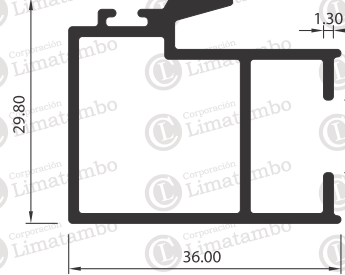
TRASLAPE DE HOJA
