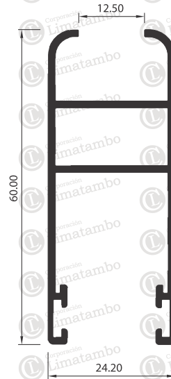
MARCO DE HOJA
