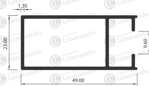
MARCO DE HOJA LATERAL
