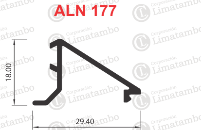
JUNQUILLO
