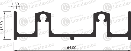
MARCO INFERIOR
