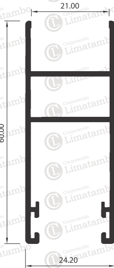
MARCO DE HOJA PARA INSULADO
