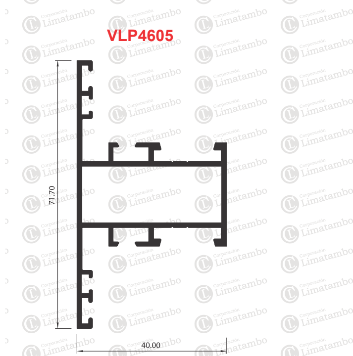
TRAVESAÑO DE VENTANA
