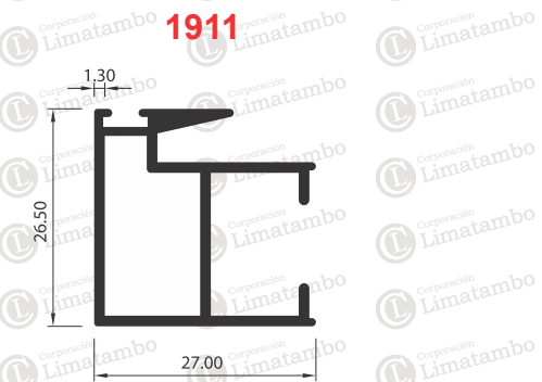
TRASLAPE
