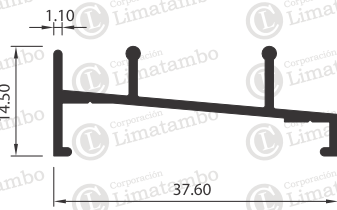
MARCO INF. DOBLE CORREDIZA
