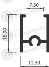
MARCO DE HOJA FIJO
