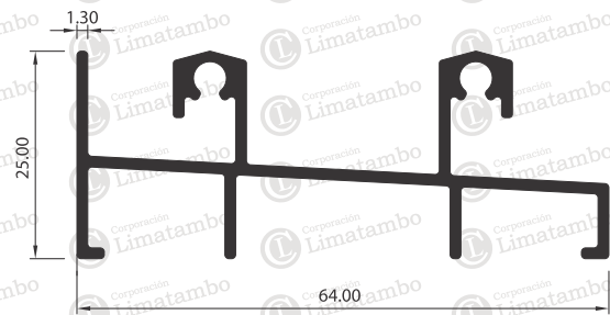
MARCO INFERIOR
