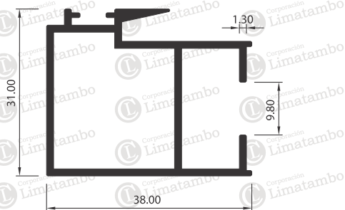
TRASLAPE
