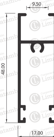
MARCO DE HOJA INFERIOR
