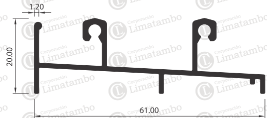
MARCO INFERIOR
