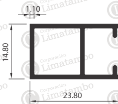
MARCO DE HOJA VERTICAL
