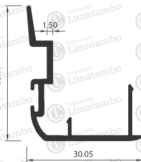
TRASLAPE
