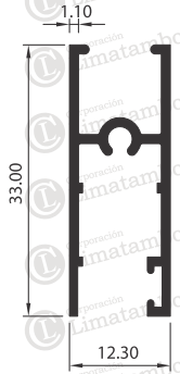
MARCO DE HOJA SUP. E INF. CORREDIZA
