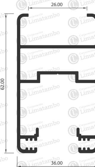
MARCO DE HOJA PARA INSULADO
