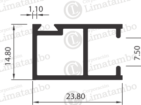
TRASLAPE DE HOJA
