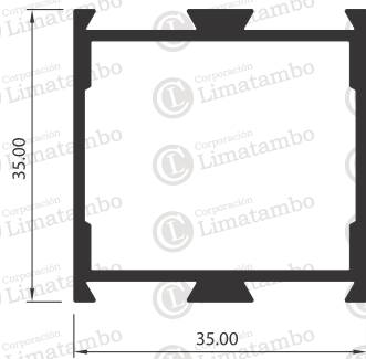
MARCO DE HOJA LIVIANA
