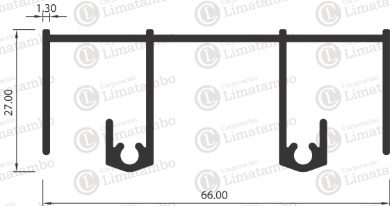
MARCO SUPERIOR
