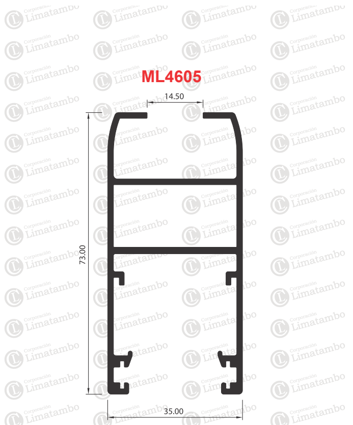
MARCO DE HOJA
