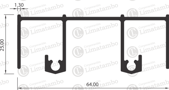
MARCO SUPERIOR
