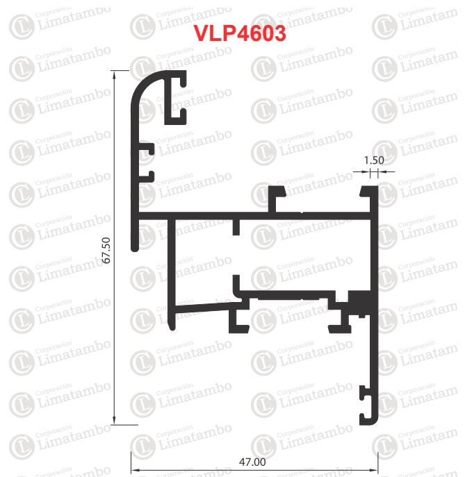
HOJA DE VENTANA APERTURA INTERIOR
