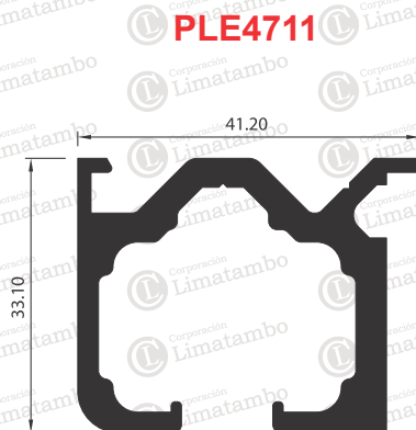
RIEL SUPERIOR PARA PLEGADIZA
