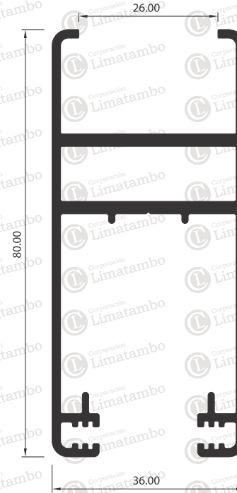
MARCO DE HOJA PARA INSULADO
