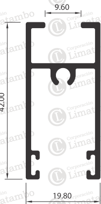
ZÓCALO DE HOJA SUPERIOR
