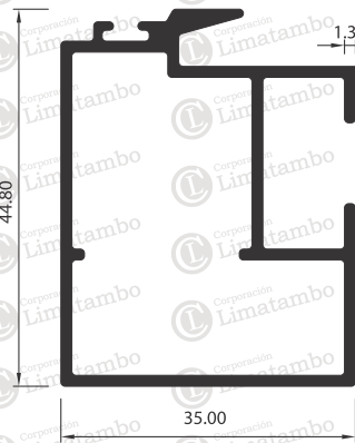
TRASLAPE DE HOJA
