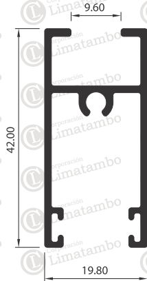
ZÓCALO DE HOJA SUPERIOR
