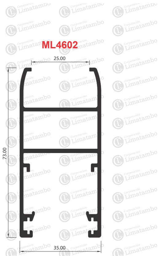
MARCO DE HOJA PARA INSULADO
