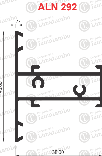
TRAVESAÑO
