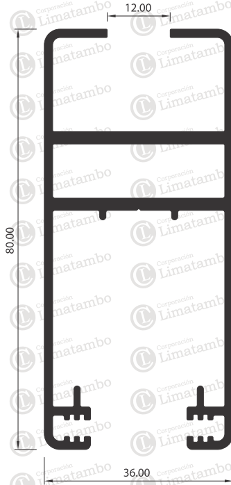
MARCO DE HOJA
