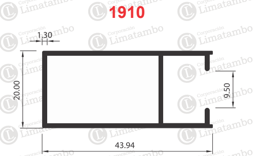
MARCO DE HOJA LATERAL
