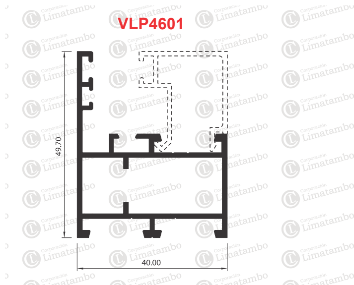
MARCO VENTANA
