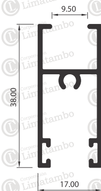
MARCO DE HOJA SUPERIOR
