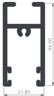
ZÓCALO SUPERIOR
