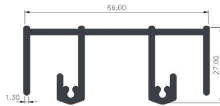
RIEL SUPERIOR
