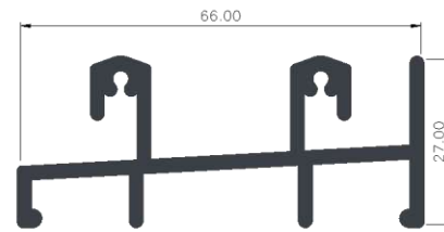
RIEL INFERIOR
