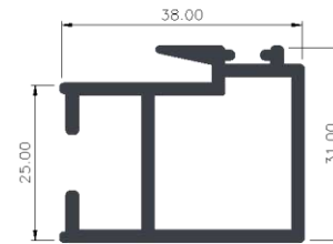
TRASLAPE
