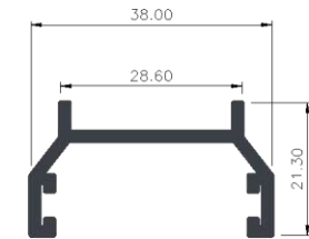
PERFIL ADAPTADOR
