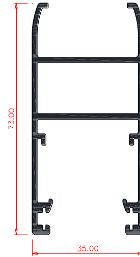
ML4602 MARCO DE HOJA INSULADO
