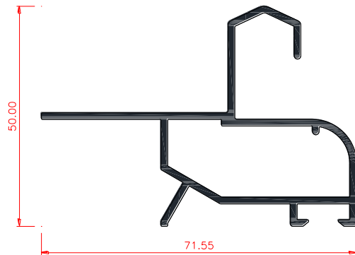
ML4604 ADAPTADOR MARCO TRIPLE CORREDIZA
