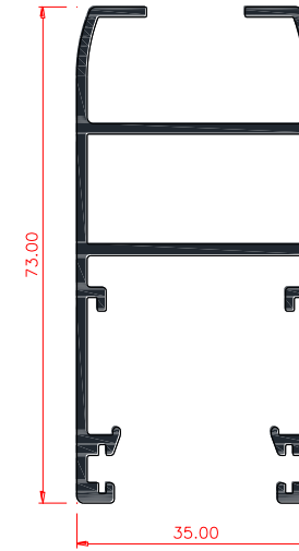
ML4605 MARCO DE HOJA
