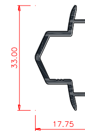
ML4606 ADAPTADOR DE HOJA
