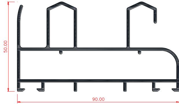
ML4601 MARCO DOBLE CORREDIZA
