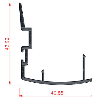
ML4603 TRASLAPE
